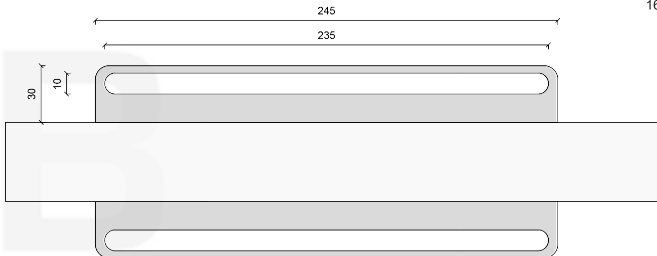
Bovenaanzicht
