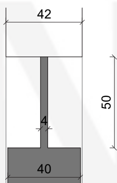
Vooraanzicht deurblad met greep - schaal 1/2
