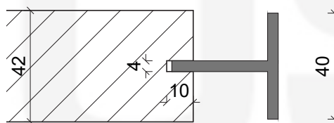
Doorsnede deurblad met greep - schaal 1/2
